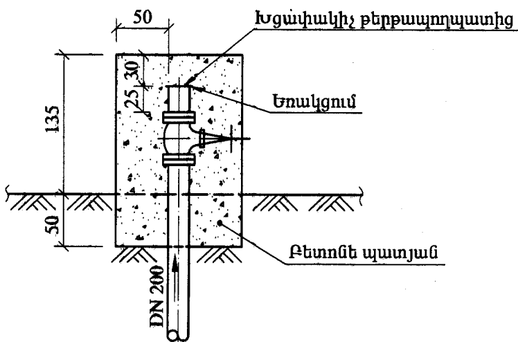
ԽՑԱՓԱԿՄԱՆ ՀԱՏԱԿԱԳԻԾԸ: Մ 1 : 50
