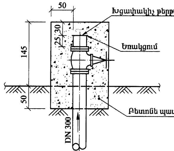
Կտրվածք 2 - 2: Մ 1 : 50
