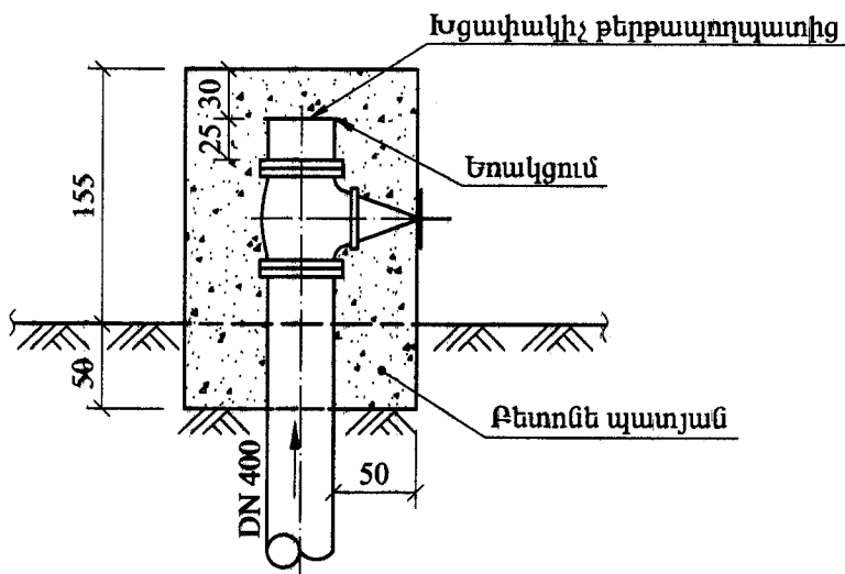
Կտրվածք 3 - 3: Մ 1 : 50
