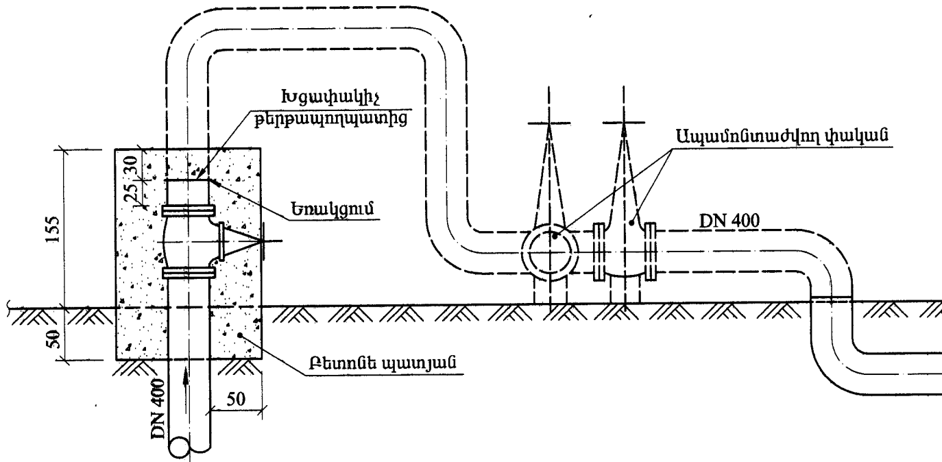
ԽՑԱՓԱԿՄԱՆ ՀԱՏԱԿԱԳԻԾԸ: Մ 1 : 50
