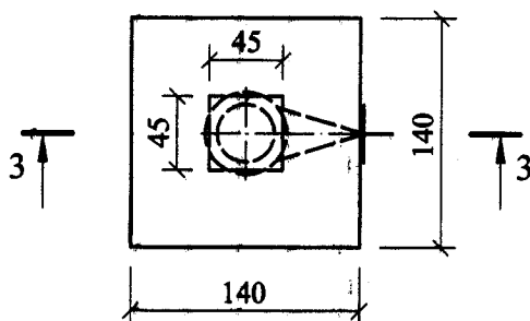
ԽՑԱՓԱԿՄԱՆ ՀԱՏԱԿԱԳԻԾԸ: Մ 1 : 50
