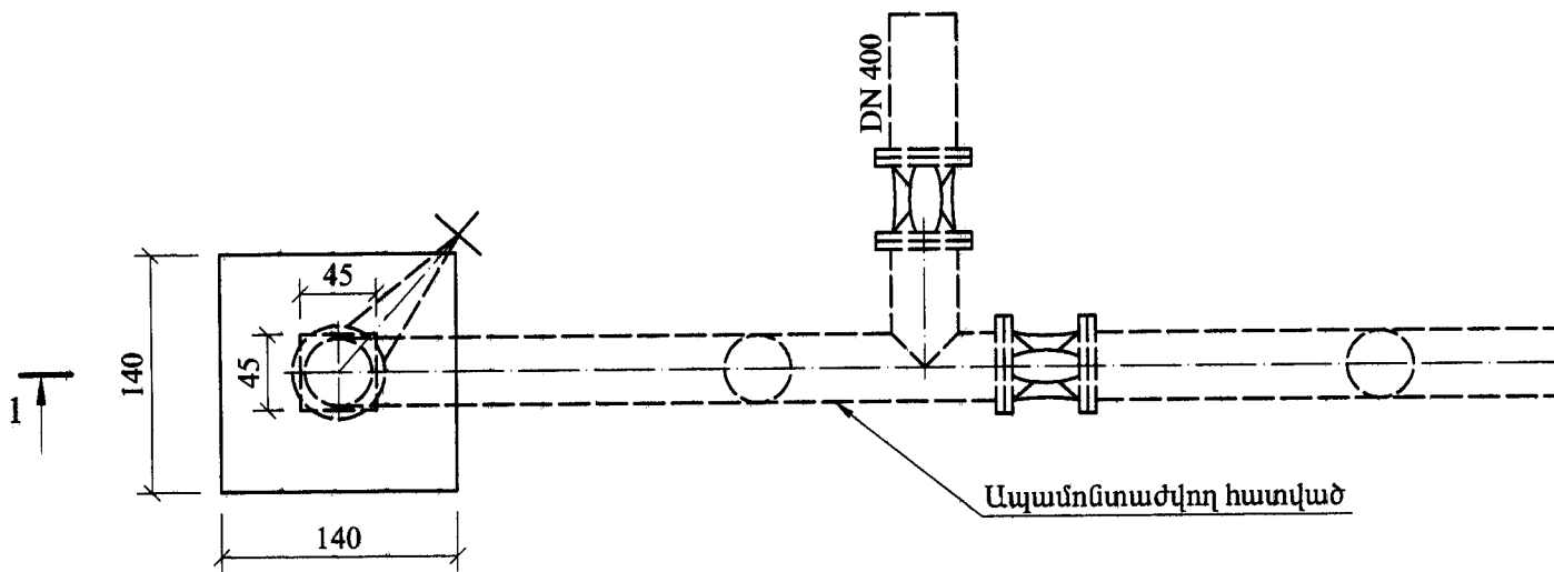
ԽՑԱՓԱԿՄԱՆ ՀԱՏԱԿԱԳԻԾԸ: Մ 1 : 50
