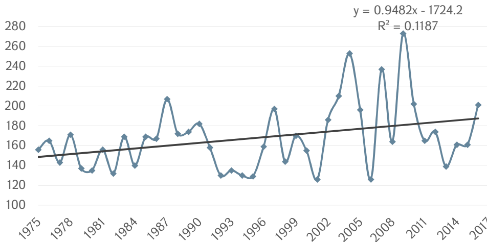
Նկար 3. Հայաստանի տարածքում 1975-2016թթ. ընթացքում դիտված վրանգավոր երևույթների՝ ցրտահարության, կարկուտի, ուժեղ քամու և առատ տեղումների գումարային դեպքերի քանակը
